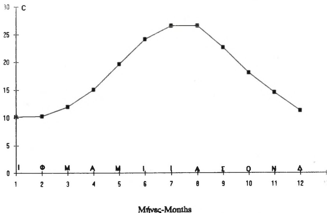
Σχήμα 1: Μέσες μηνιαίες τιμές θερμοκρασίας αέρα στην Κέρκυρα (1950-1972) Graph 1: Mean monthly air temperature in Kerkyra (1950-1972)
