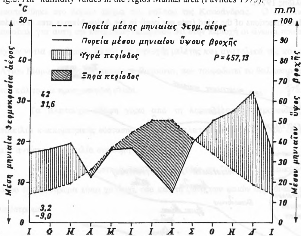
Εικ.3. Ομβροθερμικό διάγραμμα της περιοχής του Αγίου Μάμα (Παυλίδης 1975).
